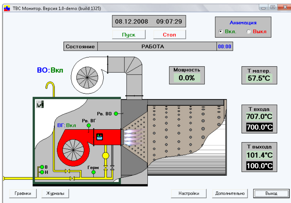
Рис. 1. Окно программы
