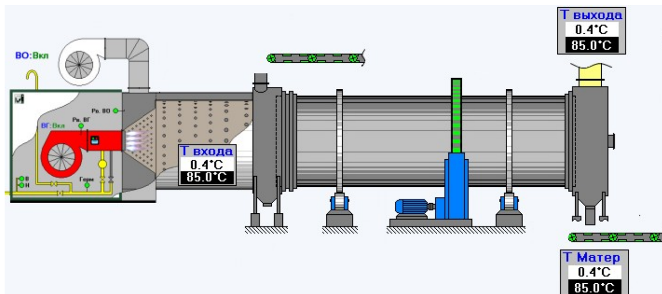
Рис.1 Расположение термодатчиков.
