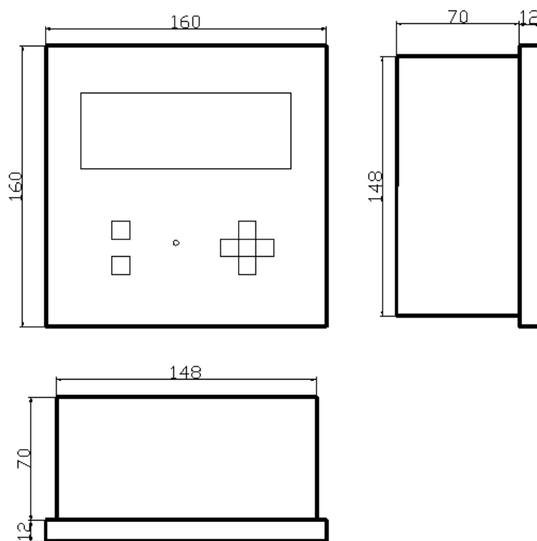
Рис.3. Блок управления ВЕГА-5.
